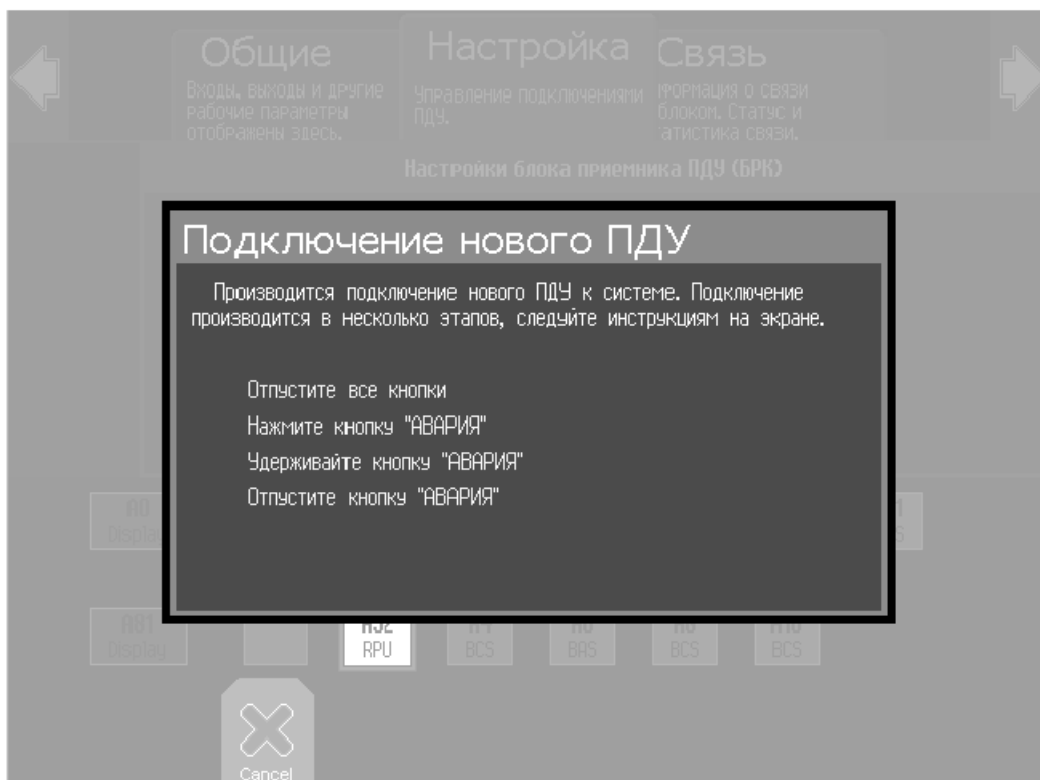
Рис. 7.10.3 – Сообщение о подключении ПДУ.
