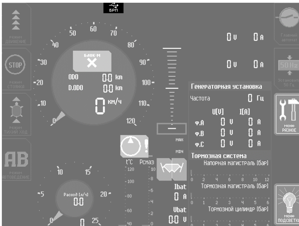
Рис. 7.9.1 – Основной экран АСКУМ с индикатором USB-флеш-накопителя
